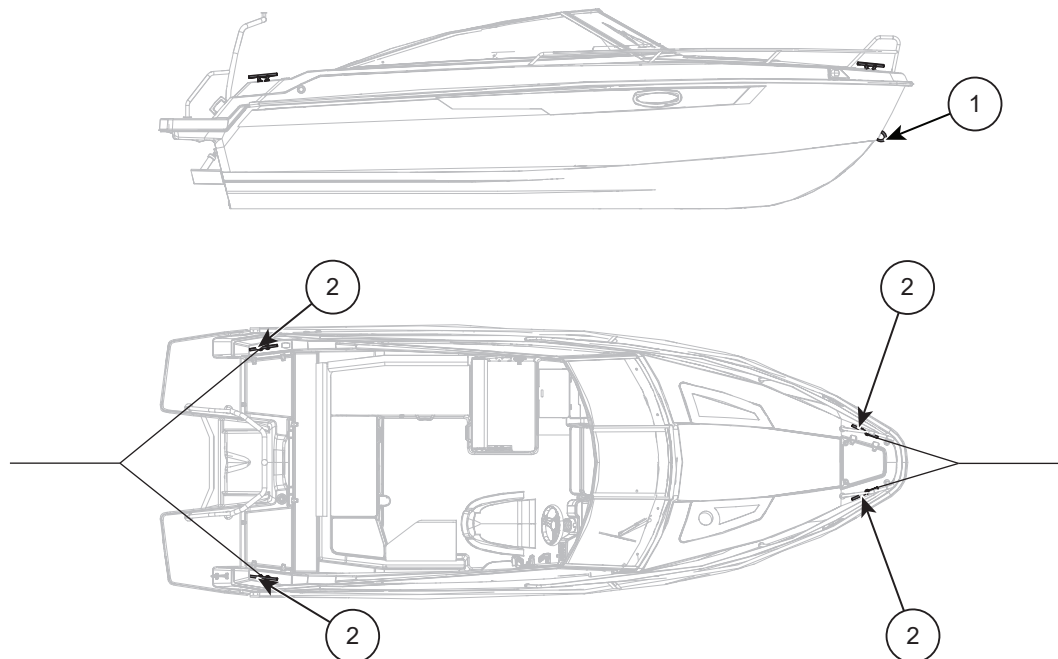
Kuva 5.7 Yamarin 63 DC kiinnitys- ja hinauspisteet
