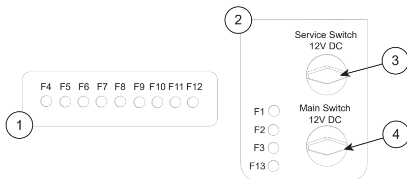
Kuva 8.1 Yamarin 63 DC/BR päävirtakytkimet ja sulakepaneeli
