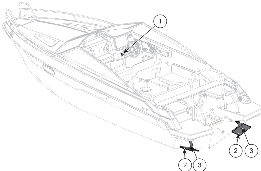
Kuva 5.6 Yamarin 63 DC trimmijärjestelmä
