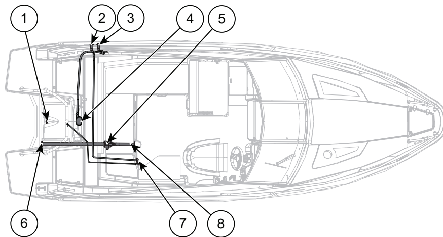
Kuva 9.1 Yamarin 63 DC pilssipumput ja tyhjennys
